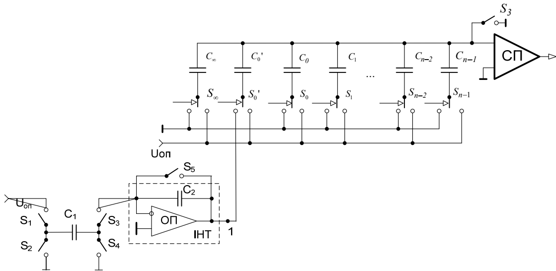
Рис. 3. Апаратна реалізація
