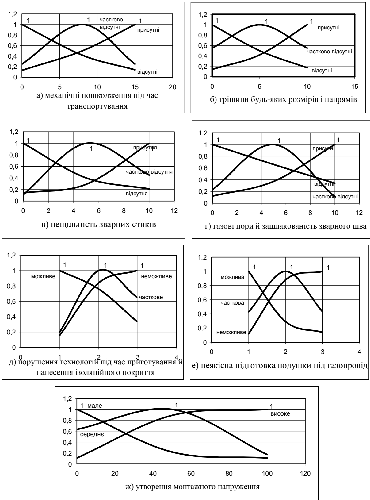
Рис. 1. Функції належності для лінгвістичних змінних, що описують будівельно-монтажні роботи Використовуючи аналітичні формули (4) – (8) та значення функцій належності змінних y_1, y_2, y_3 та y_4 (рис. 1) отримані значення функцій належності терм-оцінок змінної Y :
