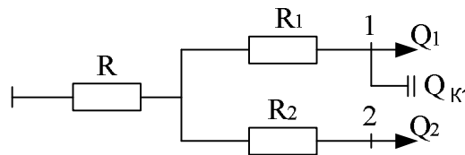
Рис. 2. Заступна схема елементарної мережі: R – значення активного опору живильної мережі; R_1, R_2 – еквівалентні активні опори мереж першої та другої частин електричної мережі; Q_1, Q_2 – реактивні навантаження відповідно першого та другого вузлів
