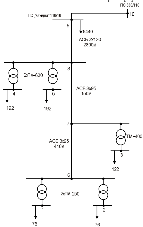
Рис. 3. Схема розрахункової мережі
