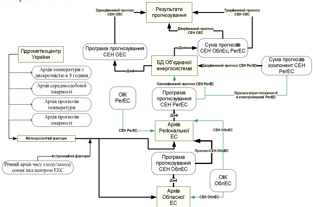
Рис. 1. Блок-схема тривіневого розв’язання задачі короткострокового прогнозування СЕН ОЕС України
