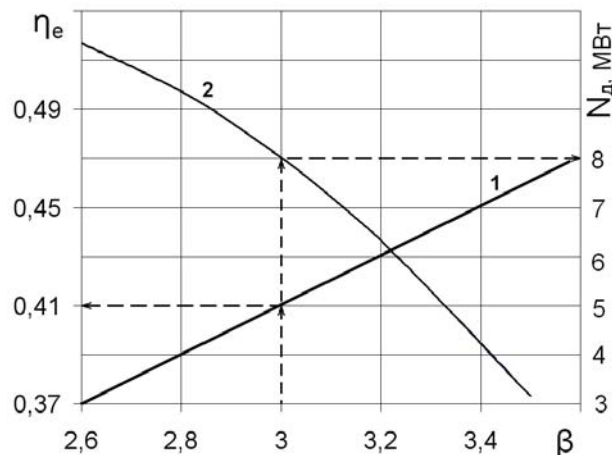
Рис. 2. Геометрична інтерпретація характеру зміни коефіцієнта використання енергії на ПАЕС і потужності ДГА: 1 – \eta_e = f(\beta) ; 2 – N_D = f_1(\beta) .
