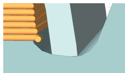
Рис. 2. а) Контакт магнітопроводу та западини колеса здійснюється по лініям дотику; б) Магнітопровід прилягає до западини повністю по всій площині
