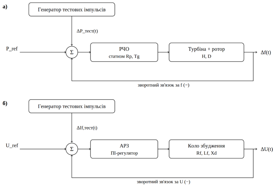
Рис. 1. Структурна схема контуру активної потужності (а) та реактивної потужності (б) з підсумовуючою ланкою для введення тестового сигналу
