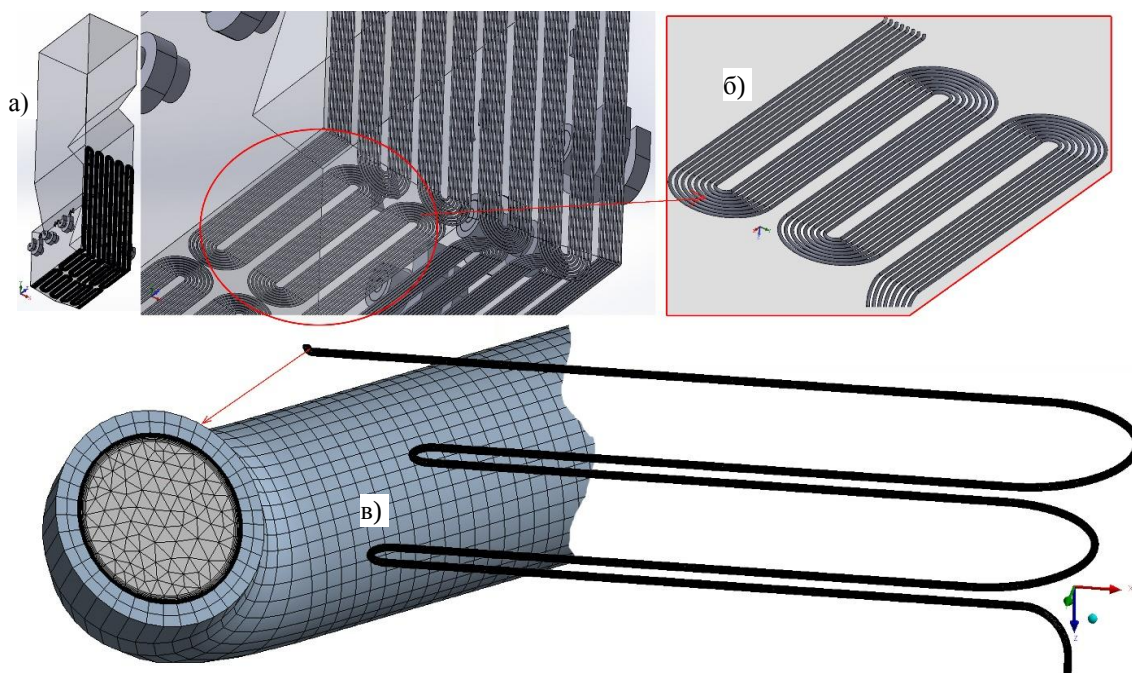
Рис. 1. Геометрична модель елементів подового екрану котла ТПП-210а та сіткова дискретизація розрахункового домену:
