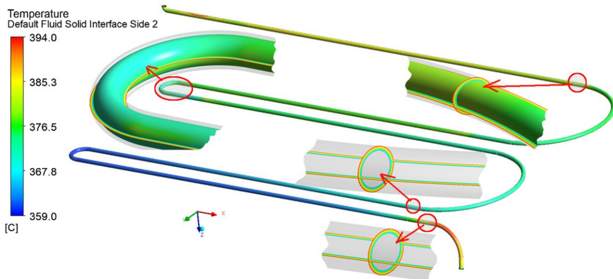
Рис. 5. Розподіл температурного поля T_w стінки подової труби та поперечні температурні градієнти.
