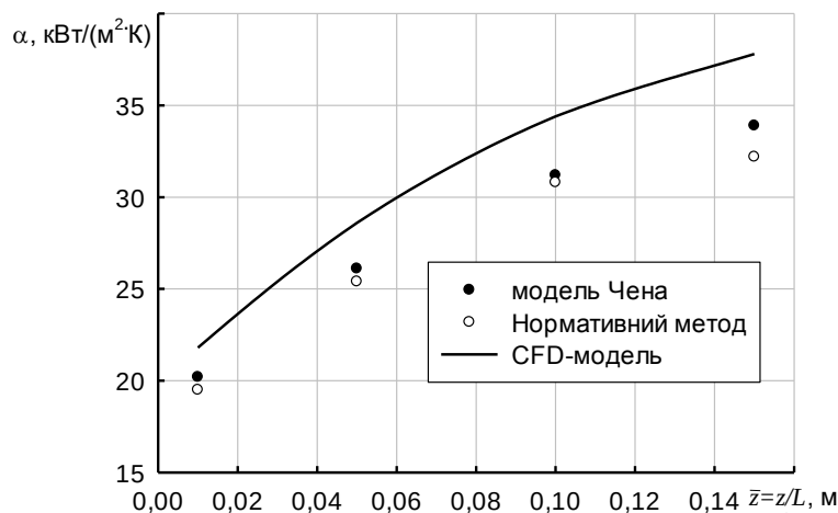
Рис. 2. Верифікація числової моделі двофазного теплообміну
