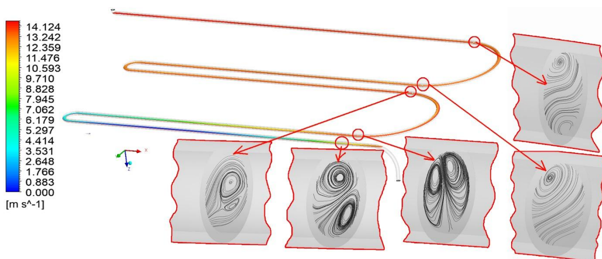
Рис. 4. Поле модуля швидкості двофазного потоку та структура вторинних течій (вихорів Діна) у поперечних перерізах подової труби та еволюція вторинних вихорних структур у перерізах 180-градусних вигинів (калачів).
