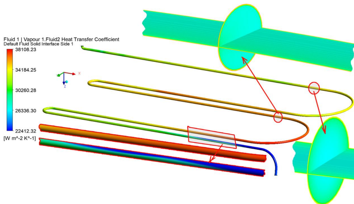
Рис. 6. Розподіл локального коефіцієнта тепловіддачі (НТС) на внутрішній поверхві подової труби.
