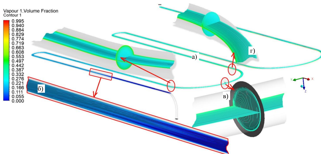
Рис. 3. Розподіл об'ємної частки парової фази \alpha_v вздовж подового змійовика котла ТПП-210а: а) загальний вигляд поля паровмісткості; б) деталізація пристінкового кипіння на вхідній ділянці; в) гравітаційне розшарування фаз на слабонахиленому каналі; г) перерозподіл двофазної суміші в 180-градусному вигині (калачі).
