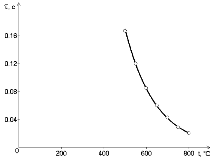
Рис. 1. Зміна часу затримки займання за збільшення температури нагрівання повітряного потоку при спалюванні біомаси: фактична \circ , теоретична —
