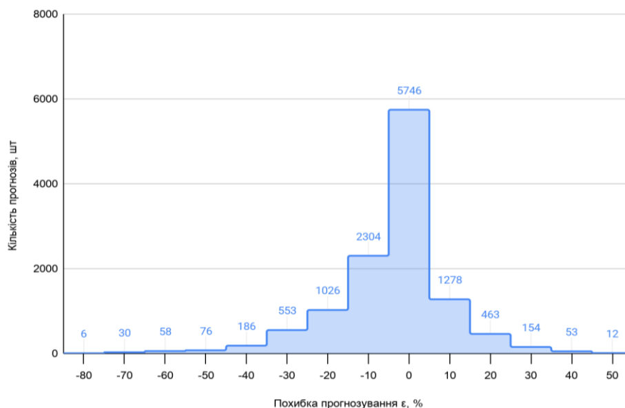
Рис. 1. Гістограма частотного розподілу похибок прогнозування агрегатора ФЕС (повна вибірка з фільтрацією)
