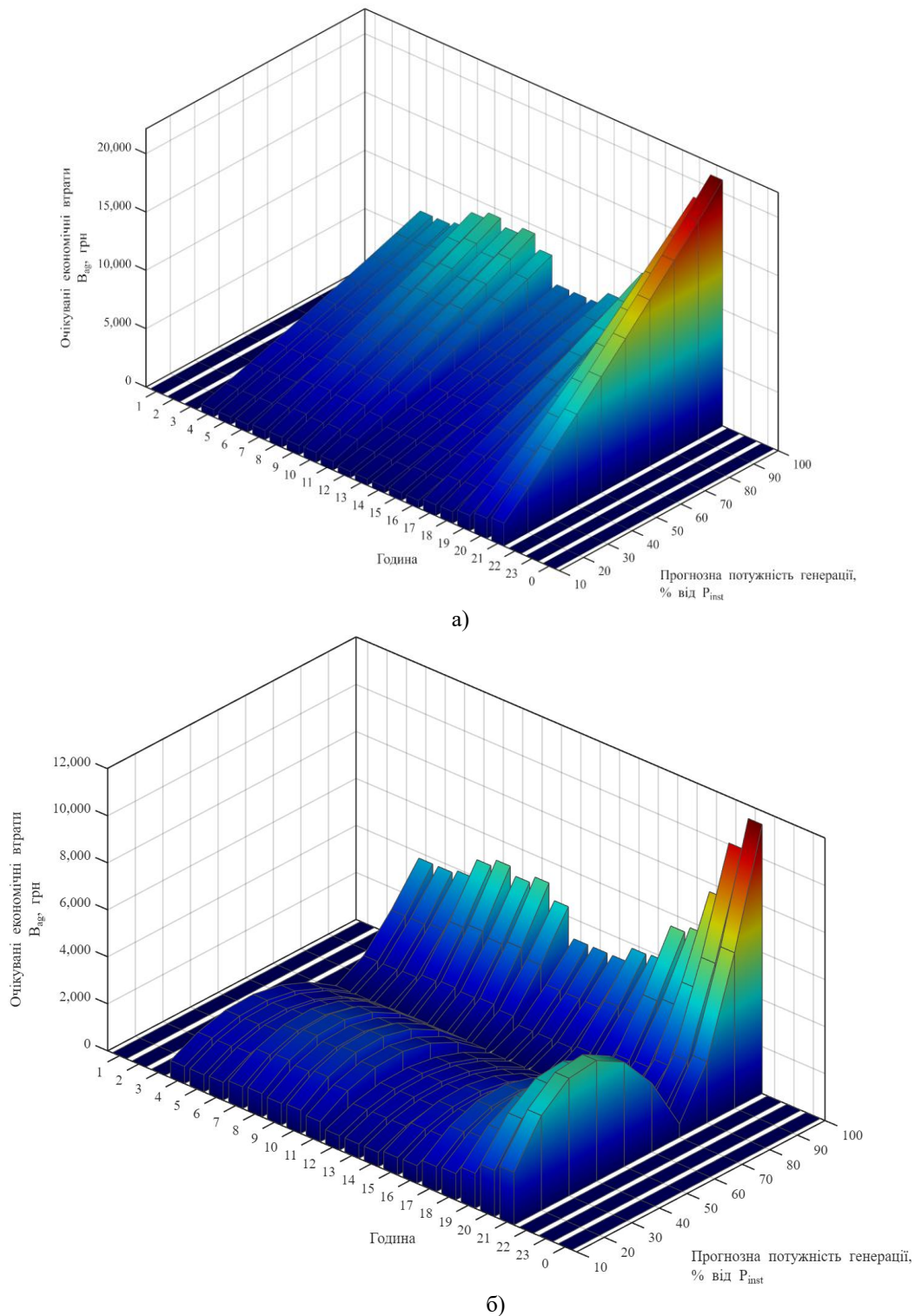
Рис. 6. Тривимірна діаграма витратної характеристики агрегатора, побудована за квантилем q_{0.05} (а), та за квантилем q_{0.95} (б) для літнього сезону
