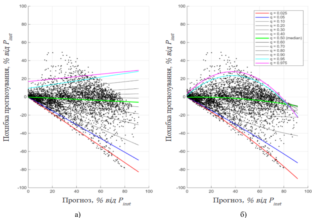
Рис. 3. Квантильні межі похибок прогнозування агрегатора ФЕС для літнього періоду: а – лінійна модель; б – квадратична модель.
