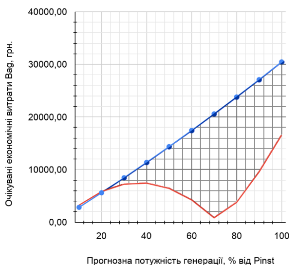
Рис. 5. Область асиметрії економічних наслідків квантильних сценаріїв похибки прогнозування
