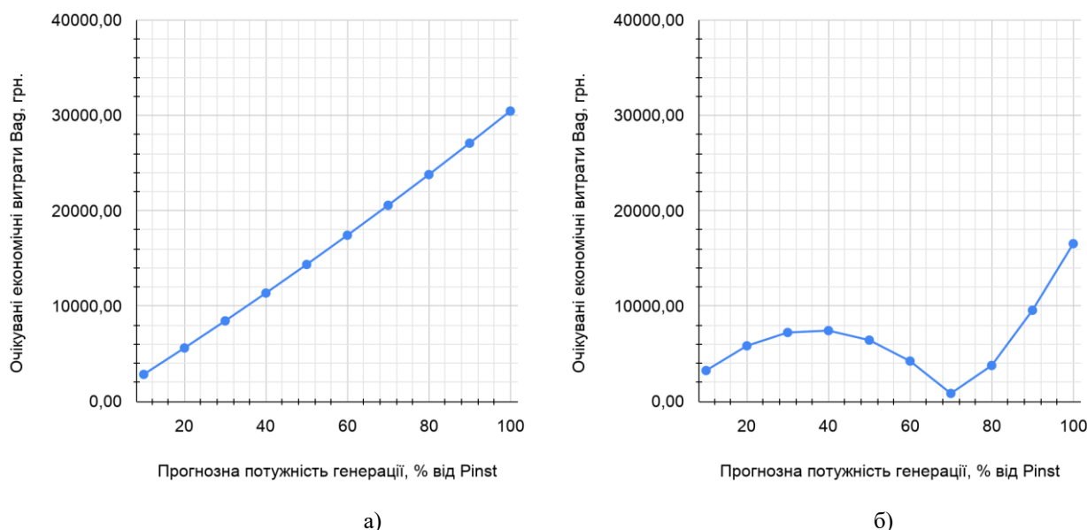
Рис 4. Витратна характеристика агрегатора для 12-ї години літнього сезону, побудована за квантилем q_{0.05} (а), та за квантилем q_{0.95} (б).
