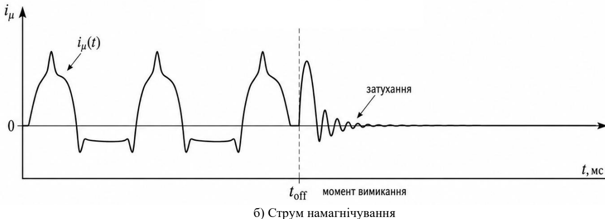
Рис. 2. Потокосцеплення та струм намагнічування під час вимкнення автотрансформатора
