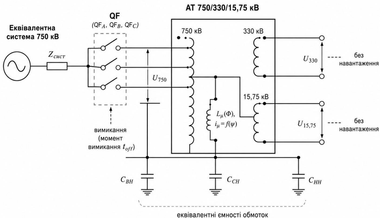
Рис. 1. Розрахункова схема вимкнення ненавантаженого автотрансформатора 750/330/15,75 кВ
