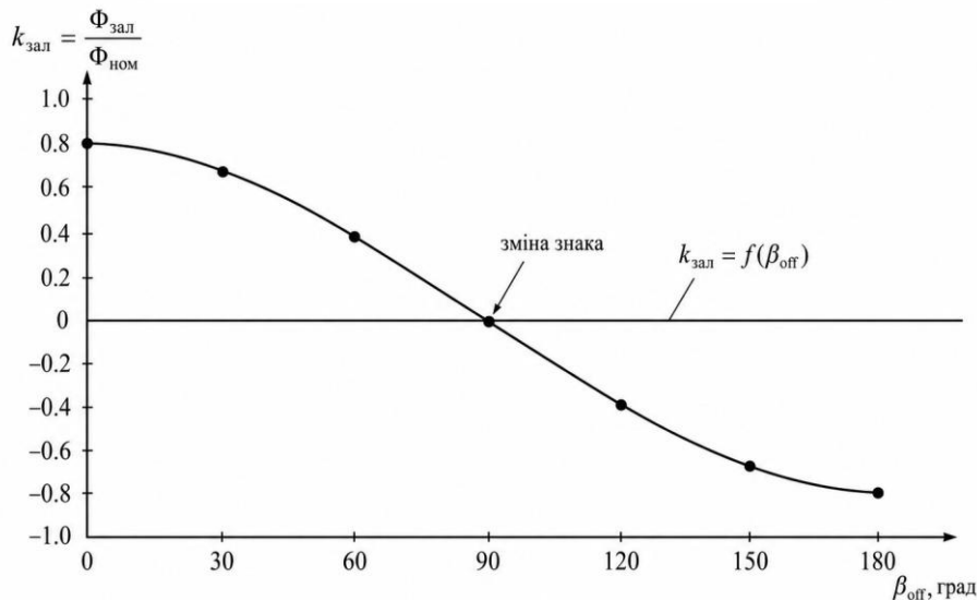
Рис. 3. Залежність залишкового магнітного потоку від кута вимкнення автотрансформатор
