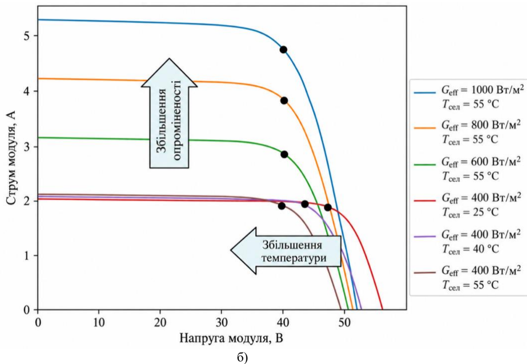
Рис. 1 Еквівалентна схема а) та ВАХ фото електричного модуля за різних значень опроміненості та температури б)
