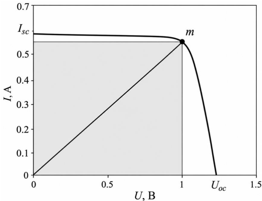
Рис. 2 Навантажувальна ВАХ фотоелектричного модуля
