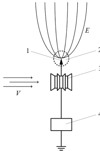
Рис. 1. Структурно-функціональна схема гібридної системи (за [18]): 1 – колектор; 2 – зона об’ємного заряду; 3 – електростатичний генератор «Дірод» із вітровим приводом; 4 – блок перетворення енергії; V – напрямок вітрового потоку; E – силові лінії атмосферного електричного поля
