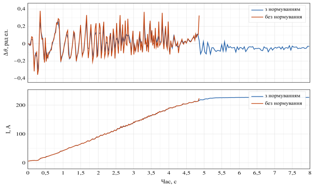
Рис. 6. Похибка оцінювання кута та амплітуда фазного струму при пуску з нормованим та класичним детектором; прогін без нормування зупинено монітором у момент передавання керування
