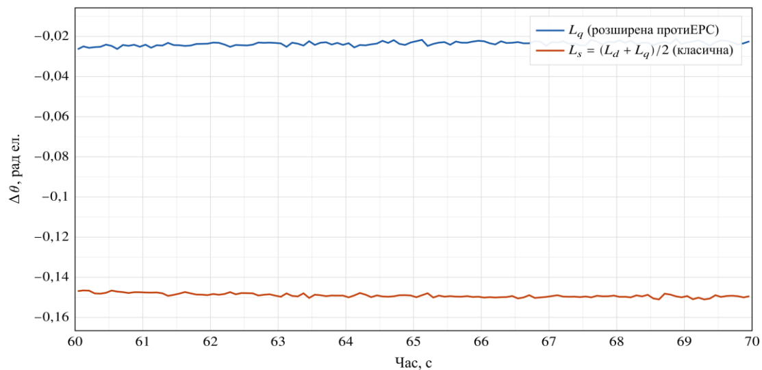
Рис. 5. Похибка оцінювання кута повороту ротора синхронного двигуна за використання L_q та середньої індуктивності L_s (усталений режим, криву згладжено)
