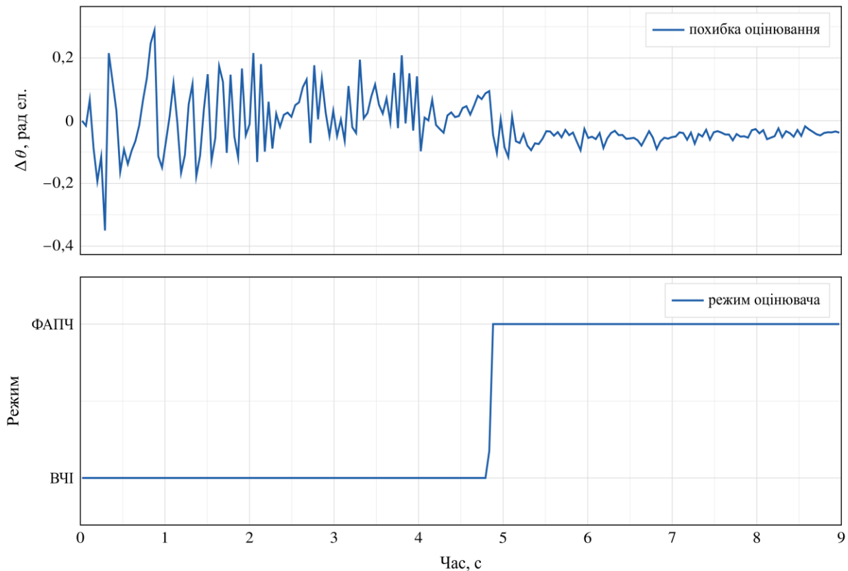
Рис. 2. Похибка оцінювання кута та режим оцінювача в циклі пуску синхронного двигуна. Криву згладжено осередненням у вікні 45 мс; показники таблиць обчислено за незгладженим рядом.
