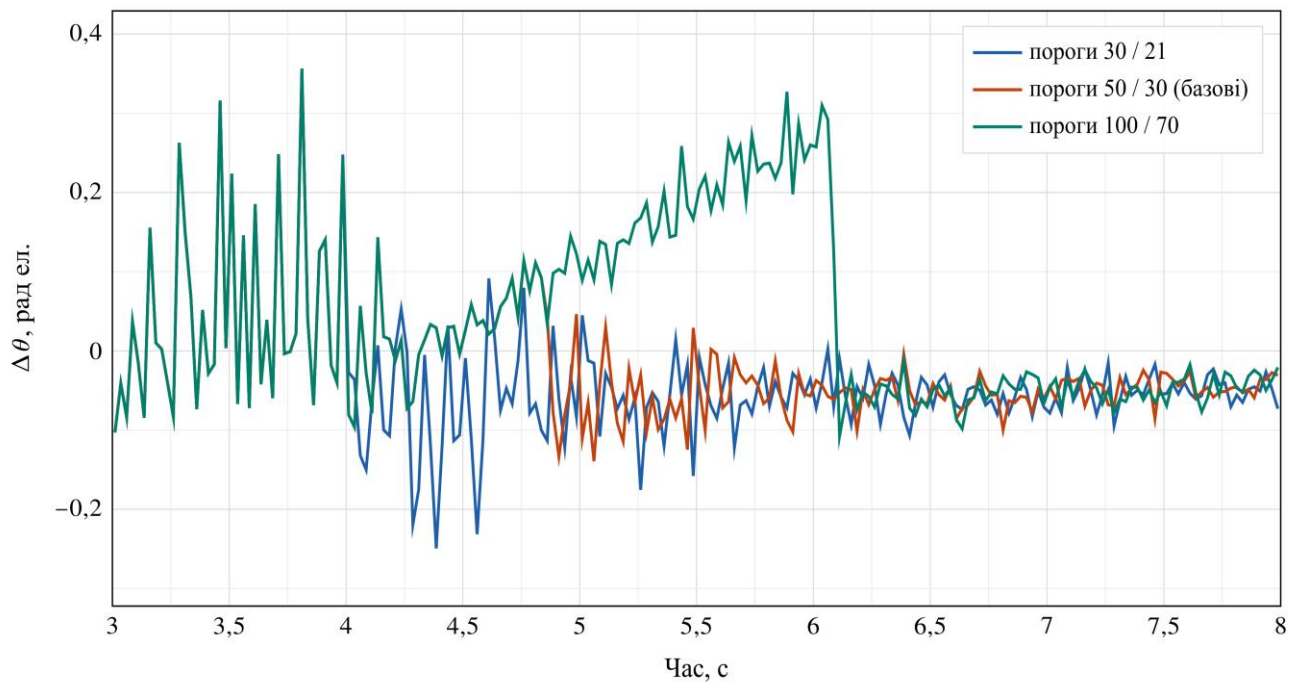
Рис. 3. Похибка оцінювання в околі передавання керування за різних порогів селектора
