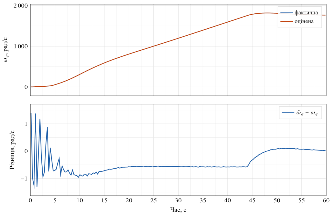
Рис. 4. Оцінена та фактична електрична кутова швидкість ротора синхронного двигуна і їх різниця
