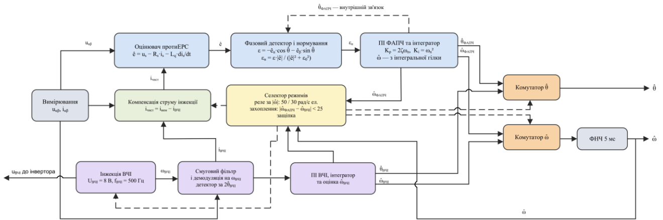
Рис. 1. Структурна схема гібридного бездавачевого спостерігача
