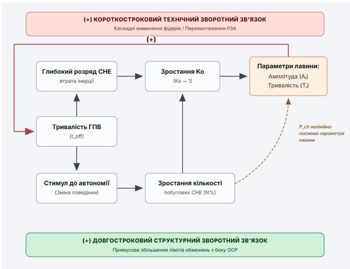
Рис. 1. Структурна схема дестабілізуючих контурів позитивного зворотного зв'язку в розподільчих мережах при застосуванні ГПВ
