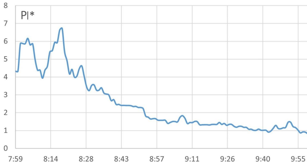
Рис. 2. Крива активної потужності споживчого вузла при «зарядній лавині»
