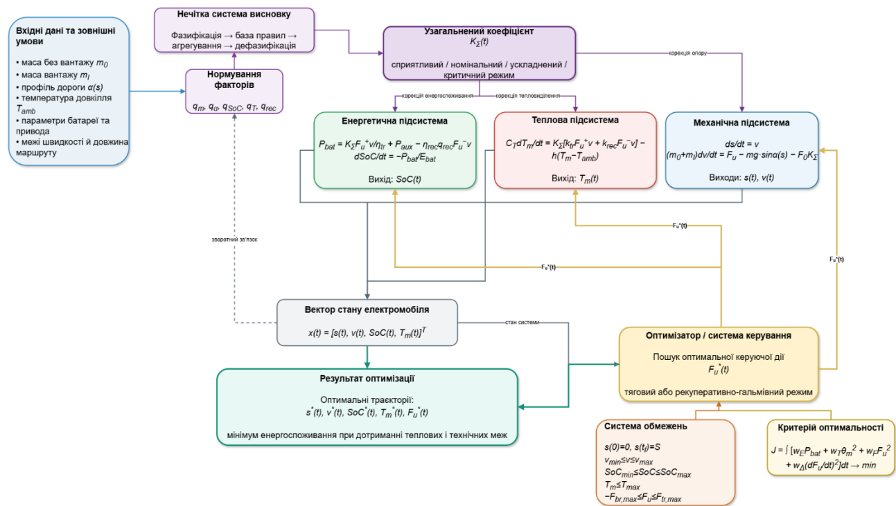
Рис. 1. Структурна схема удосконаленої математичної моделі оптимального руху завантаженого електромобіля
