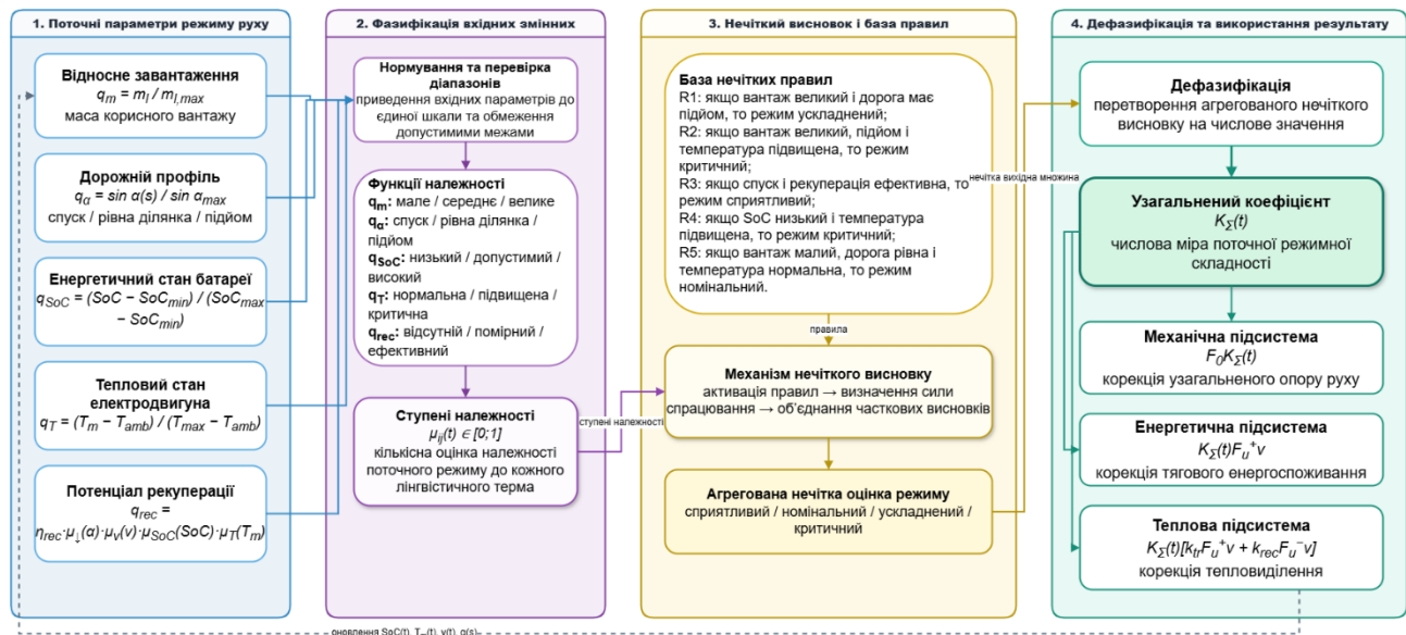
Рис. 2. Схема формування узагальненого нечіткого коефіцієнта режимної складності K_\Sigma(t)
