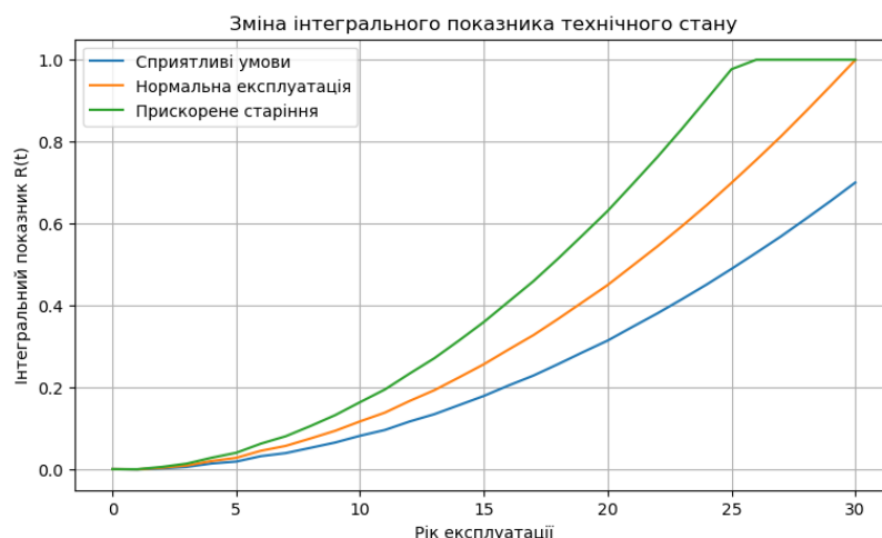
Рис. 1. Зміна інтегрального показника технічного стану R(t) , для різних сценаріїв експлуатації
