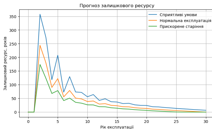
Рис. 2. Зміна прогнозованого залишкового ресурсу залежно від часу експлуатації
